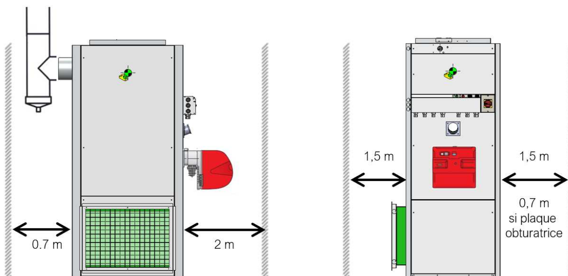
Distance minimum à prévoir autour du générateur (aucun objet ne doit se trouver à l'intérieur de ce périmètre)
