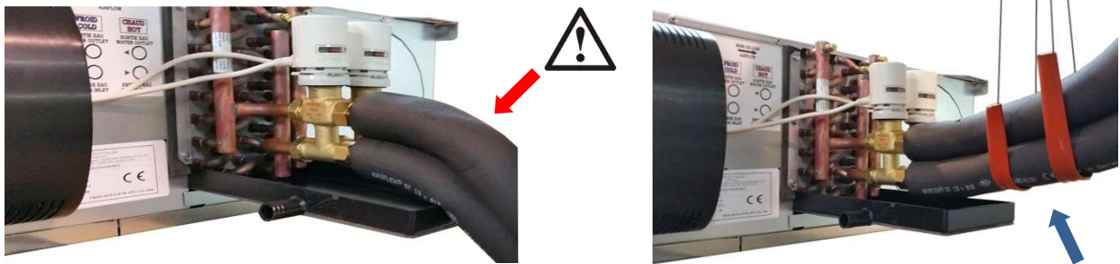
Vues indicatives d'un ventilo-convecteur FUN, la situation est identique dans le cas d'une cassette BORA.
