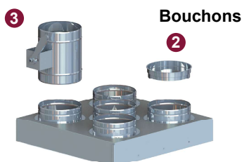
Clapet de dosage (hauteur 252 mm)
